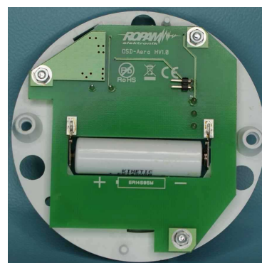
Widok czujki z modulem Aero (góra):
