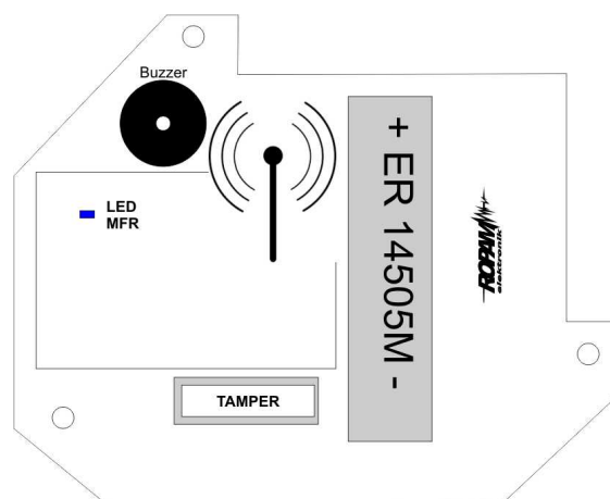
Widok ogólny czujki:
