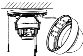
Przymocuj podstawę montażową do sufitu
